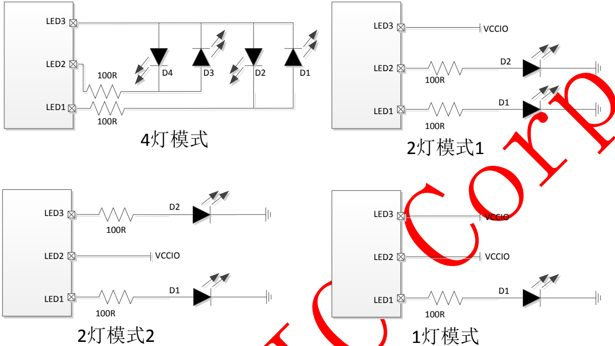
4、2、1 LED 连接方式
