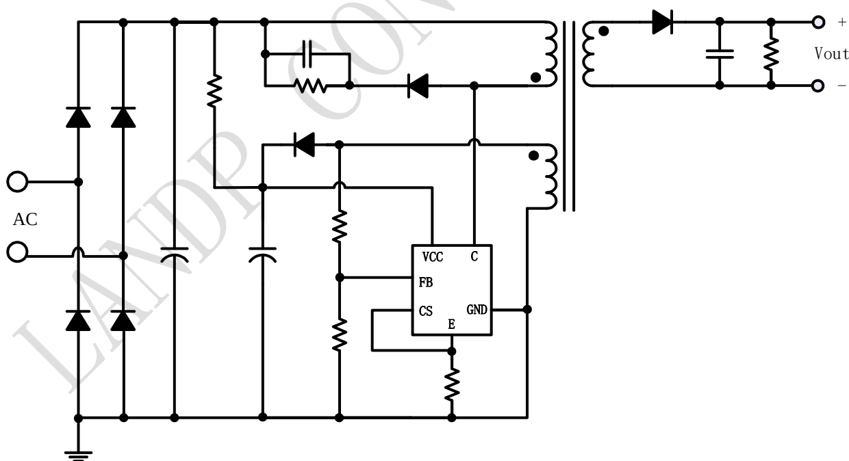
图 1 LP3773C 典型应用图
